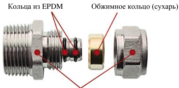
Корпус и накидная гайка из никелированной латуни CW617N
